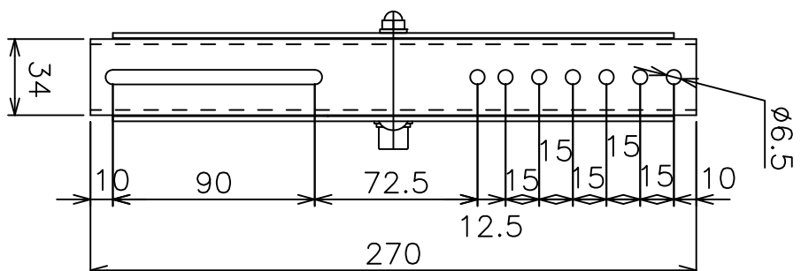
タッチメント穴位置図
