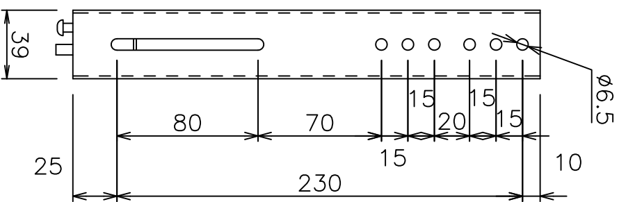
タッチメント穴位置図
