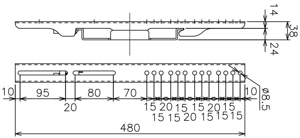
フタツチメント穴位置図
