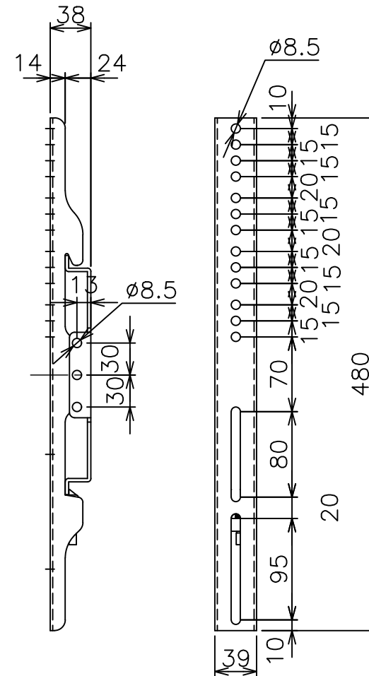
アタッチメント穴位置図
