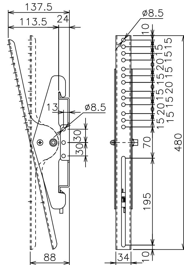
アタッチメント穴位置図
